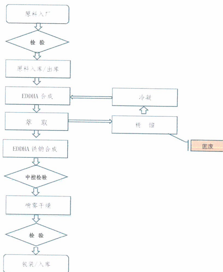
EDDHA 铁钠 工艺流程图
